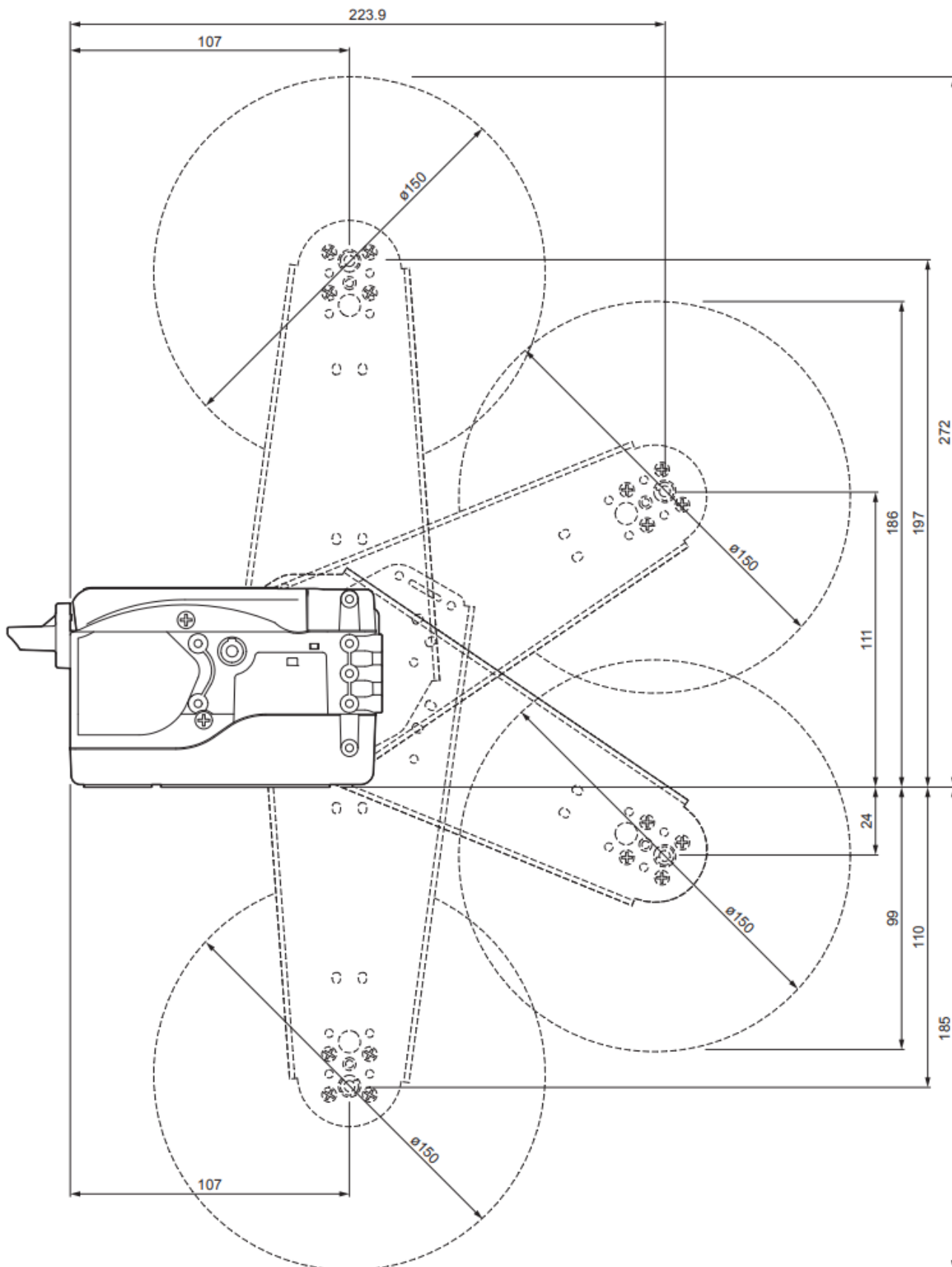
VKP80III-ФА Размеры
